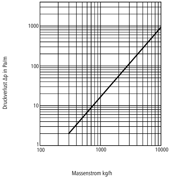
Druckverlustdiagramm Anschluss 1.1
