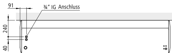
Draufsicht
