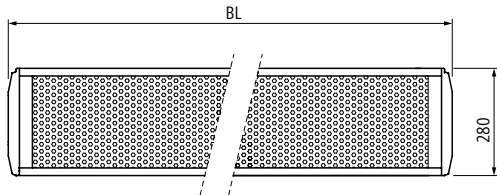
Vorderansicht
