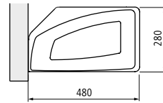
Seitenansicht
